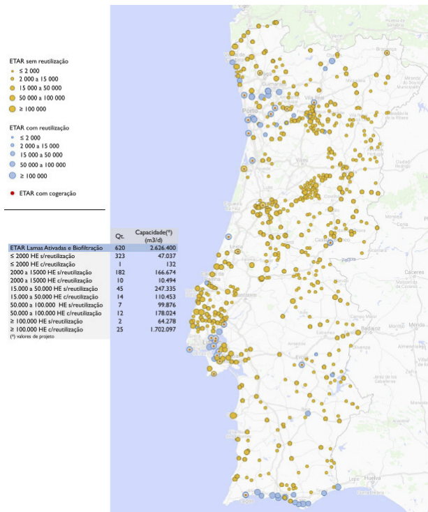
Figura 17 — Estações de Tratamento de Águas Residuais com tratamento por lamas ativadas (consideradas como as de maior potencial de sinergia com projetos H2) [Fonte: Águas de Portugal, S. A.]
